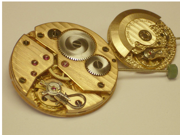
Das ETA 6497-1 und das ETA 2824 -2 kompl. Veredelt.
